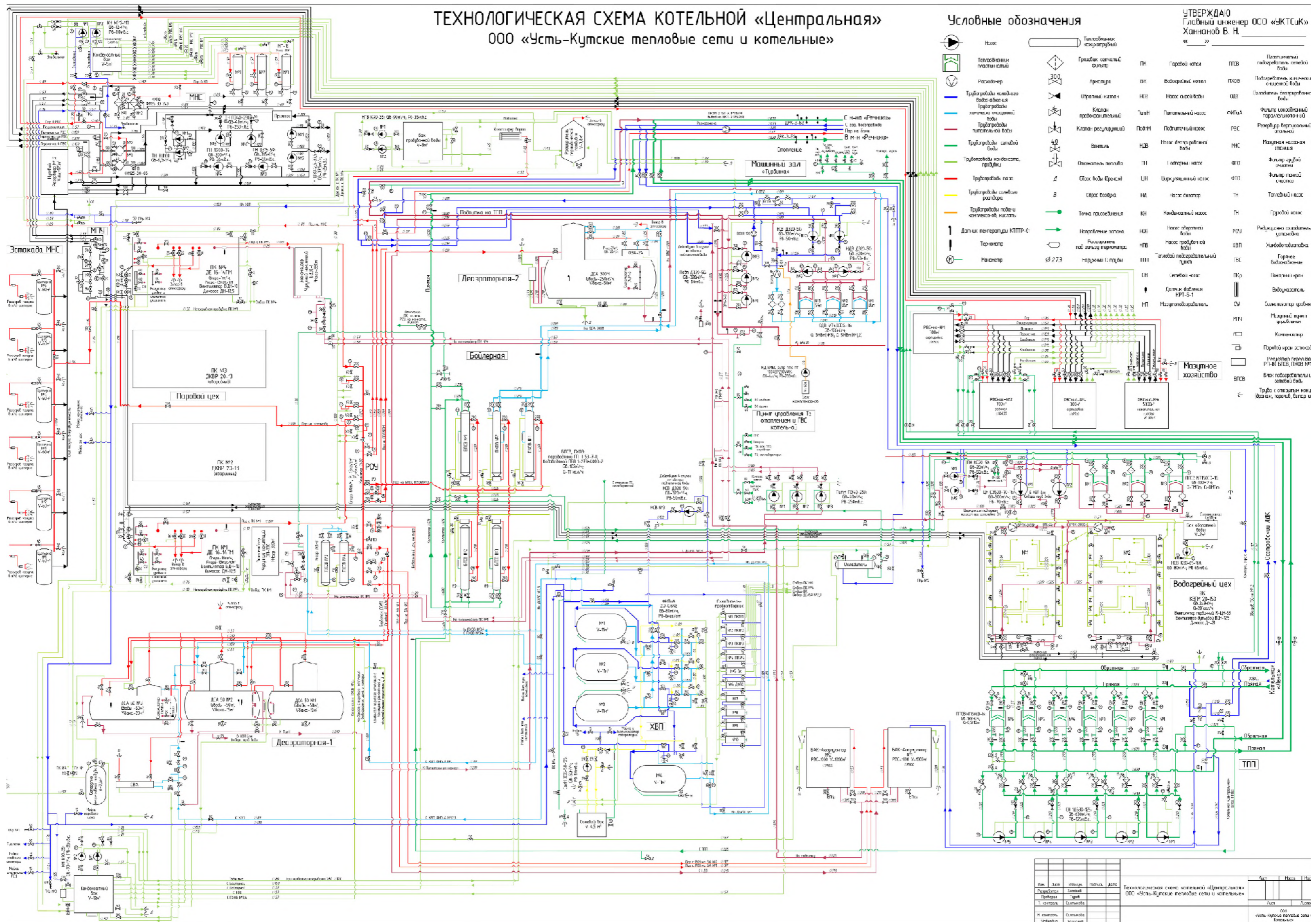
Рис. 2.3. Технологическая схема котельной «Центральная»
